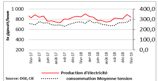
Graphique 1: Production et consommation d'électricité
